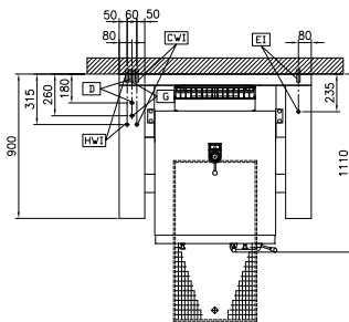
Boven aanzicht
